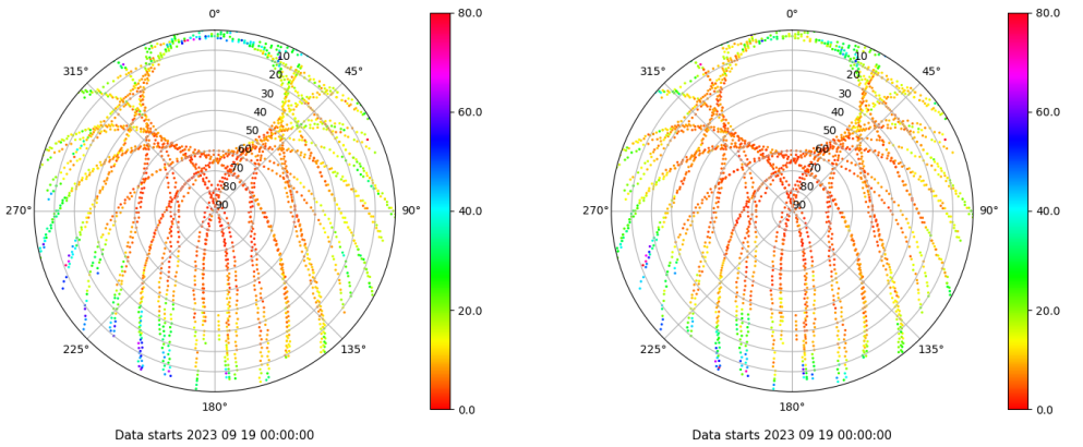
Skyplot for station XIXO. Parameter M1C Data file XIXO00ESP_R_2023262.xtr Skyplot for station XIXO. Parameter M2C Data file XIXO00ESP_R_2023262.xtr
