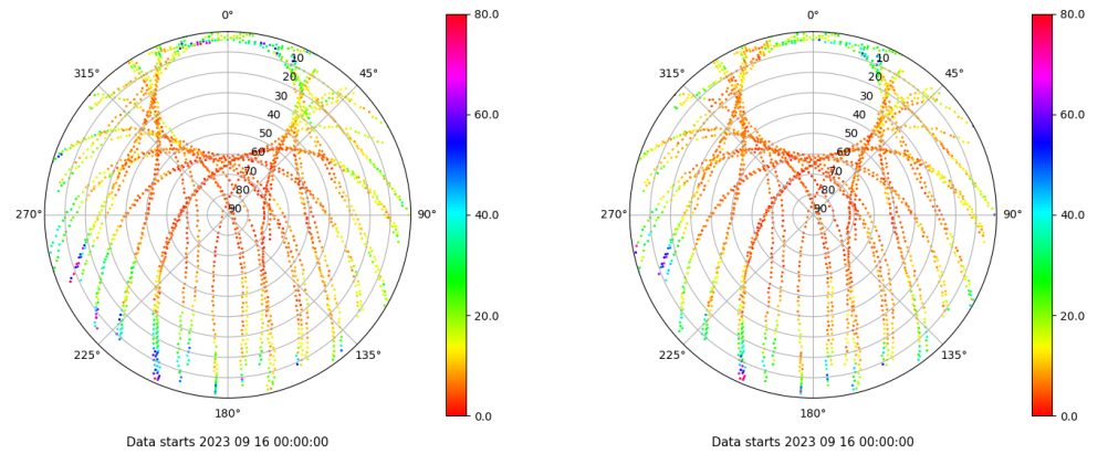
Skyplot for station XIXO. Parameter M1C Data file XIXO00ESP_R_2023259.xtr Skyplot for station XIXO. Parameter M2C Data file XIXO00ESP_R_2023259.xtr
