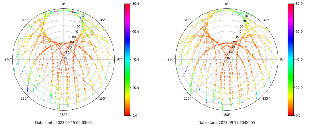
Skyplot for station XIXO. Parameter M1C Data file XIXO00ESP_R_2023258.xtr Skyplot for station XIXO. Parameter M2C Data file XIXO00ESP_R_2023258.xtr
