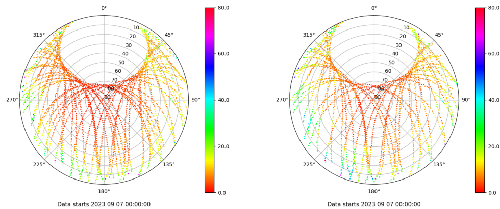
Skyplot for station XIXO. Parameter M1C Data file XIXO00ESP_R_2023250.xtr Skyplot for station XIXO. Parameter M2S Data file XIXO00ESP_R_2023250.xtr
