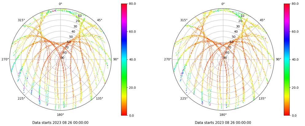
Skyplot for station XIXO. Parameter M1C Data file XIXO00ESP_R_2023238.xtr Skyplot for station XIXO. Parameter M2C Data file XIXO00ESP_R_2023238.xtr
