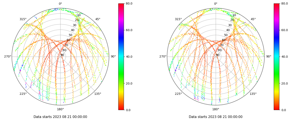
Skyplot for station XIXO. Parameter M1C Data file XIXO00ESP_R_2023233.xtr Skyplot for station XIXO. Parameter M2C Data file XIXO00ESP_R_2023233.xtr
