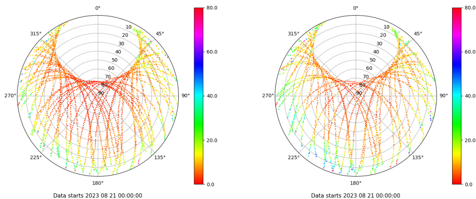
Skyplot for station XIXO. Parameter M1C Data file XIXO00ESP_R_2023233.xtr Skyplot for station XIXO. Parameter M2S Data file XIXO00ESP_R_2023233.xtr
