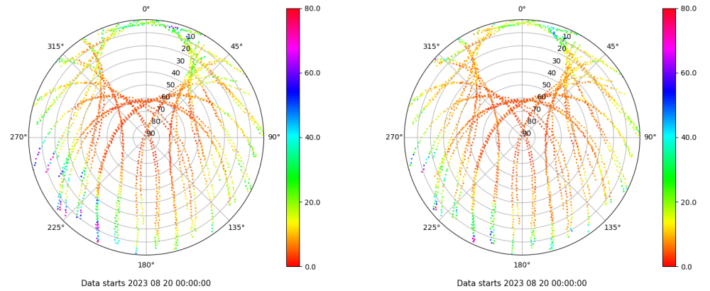
Skyplot for station XIXO. Parameter M1C Data file XIXO00ESP_R_2023232.xtr Skyplot for station XIXO. Parameter M2C Data file XIXO00ESP_R_2023232.xtr
