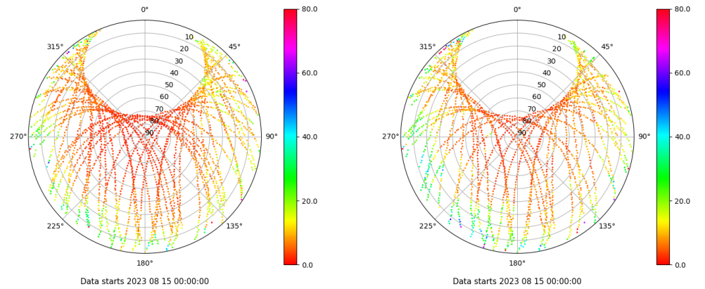
Skyplot for station XIXO. Parameter M1C Data file XIXO00ESP_R_2023227.xtr Skyplot for station XIXO. Parameter M2S Data file XIXO00ESP_R_2023227.xtr
