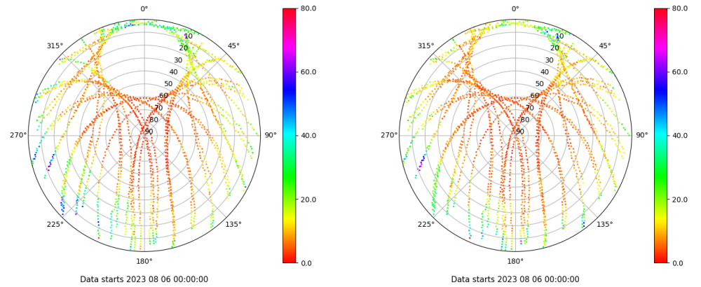
Skyplot for station XIXO. Parameter M1C Data file XIXO00ESP_R_2023218.xtr Skyplot for station XIXO. Parameter M2C Data file XIXO00ESP_R_2023218.xtr
