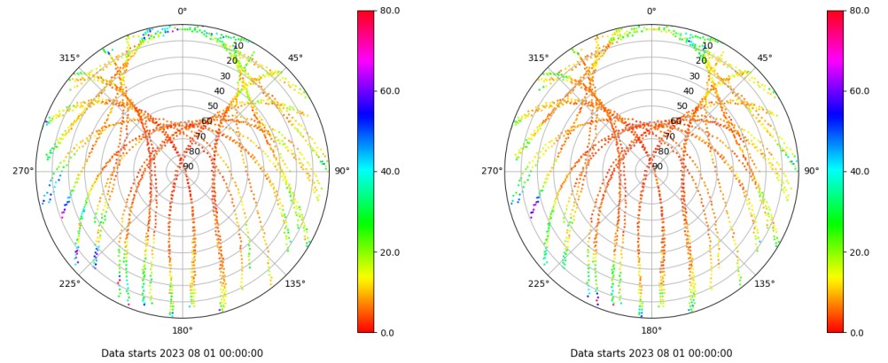
Skyplot for station XIXO. Parameter M1C Data file XIXO00ESP_R_2023213.xtr Skyplot for station XIXO. Parameter M2C Data file XIXO00ESP_R_2023213.xtr
