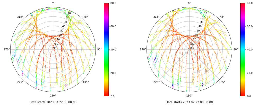
Skyplot for station XIXO. Parameter M1C Data file XIXO00ESP_R_2023203.xtr Skyplot for station XIXO. Parameter M2C Data file XIXO00ESP_R_2023203.xtr
