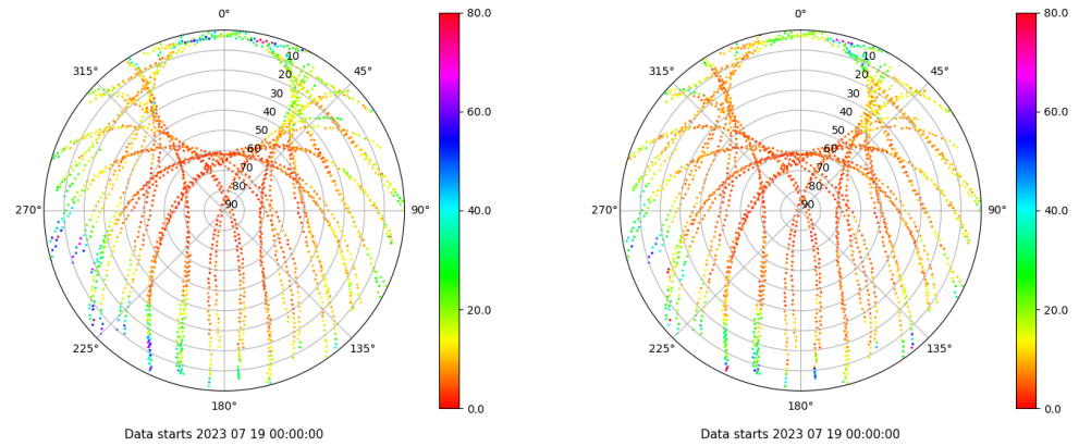
Skyplot for station XIXO. Parameter M1C Data file XIXO00ESP_R_2023200.xtr Skyplot for station XIXO. Parameter M2C Data file XIXO00ESP_R_2023200.xtr
