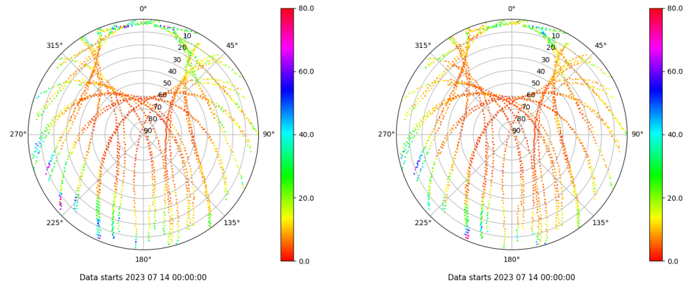
Skyplot for station XIXO. Parameter M1C Data file XIXO00ESP_R_2023195.xtr Skyplot for station XIXO. Parameter M2C Data file XIXO00ESP_R_2023195.xtr
