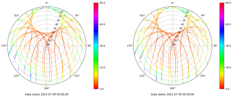
Skyplot for station XIXO. Parameter M1C Data file XIXO00ESP_R_2023190.xtr Skyplot for station XIXO. Parameter M2C Data file XIXO00ESP_R_2023190.xtr
