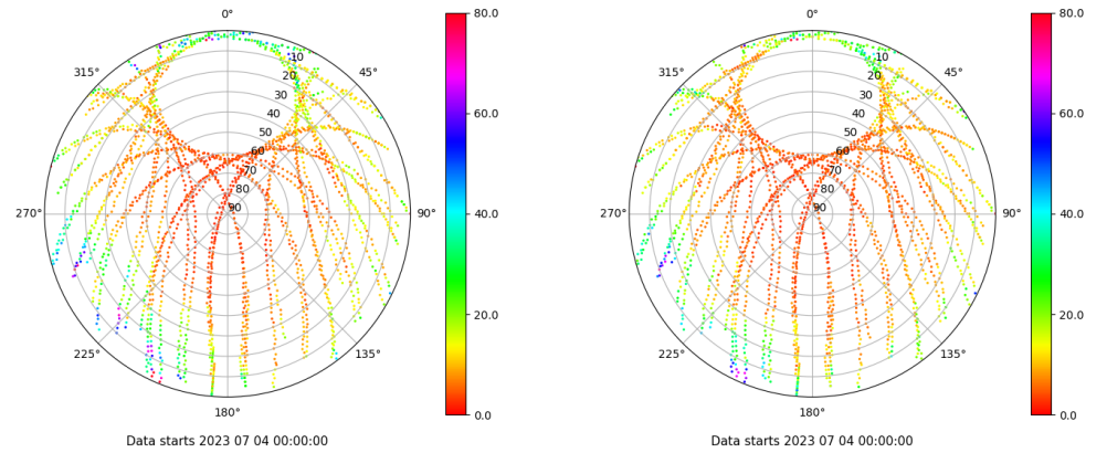
Skyplot for station XIXO. Parameter M1C Data file XIXO00ESP_R_2023185.xtr Skyplot for station XIXO. Parameter M2C Data file XIXO00ESP_R_2023185.xtr
