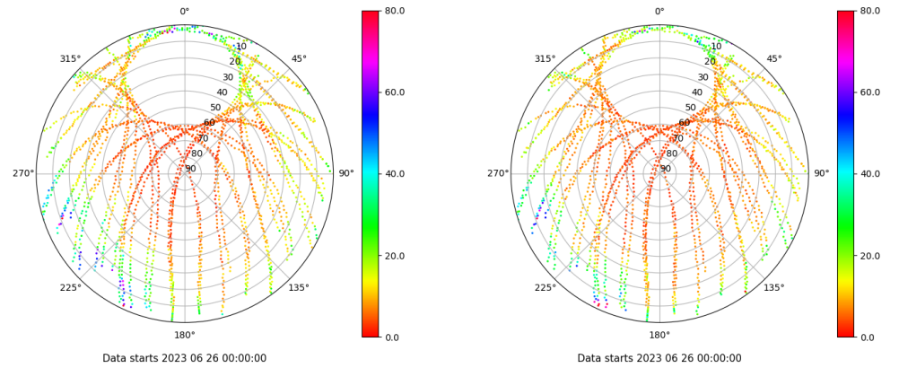
Skyplot for station XIXO. Parameter M1C Data file XIXO00ESP_R_2023177.xtr Skyplot for station XIXO. Parameter M2C Data file XIXO00ESP_R_2023177.xtr
