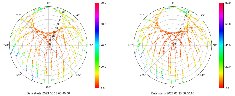
Skyplot for station XIXO. Parameter M1C Data file XIXO00ESP_R_2023174.xtr Skyplot for station XIXO. Parameter M2C Data file XIXO00ESP_R_2023174.xtr
