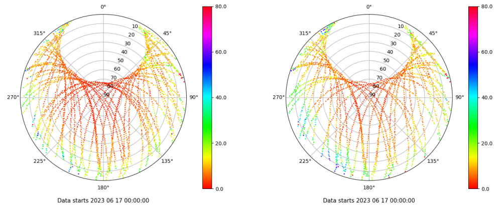
Skyplot for station XIXO. Parameter M1C Data file XIXO00ESP_R_2023168.xtr Skyplot for station XIXO. Parameter M2S Data file XIXO00ESP_R_2023168.xtr
