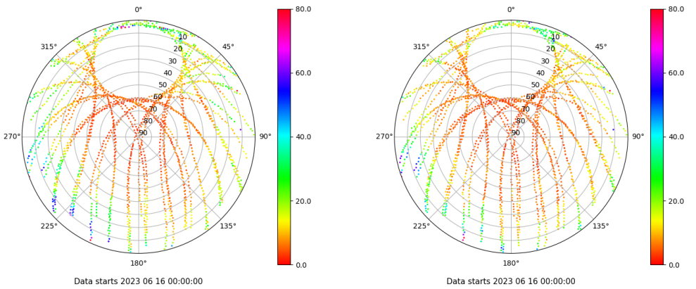
Skyplot for station XIXO. Parameter M1C Data file XIXO00ESP_R_2023167.xtr Skyplot for station XIXO. Parameter M2C Data file XIXO00ESP_R_2023167.xtr
