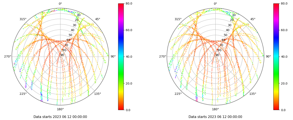
Skyplot for station XIXO. Parameter M1C Data file XIXO00ESP_R_2023163.xtr Skyplot for station XIXO. Parameter M2C Data file XIXO00ESP_R_2023163.xtr
