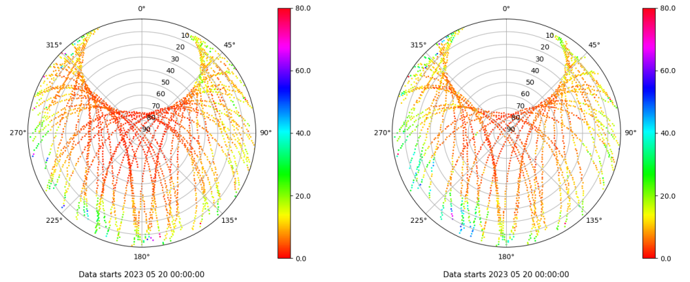
Skyplot for station XIXO. Parameter M1C Data file XIXO00ESP_R_2023140.xtr Skyplot for station XIXO. Parameter M2S Data file XIXO00ESP_R_2023140.xtr
