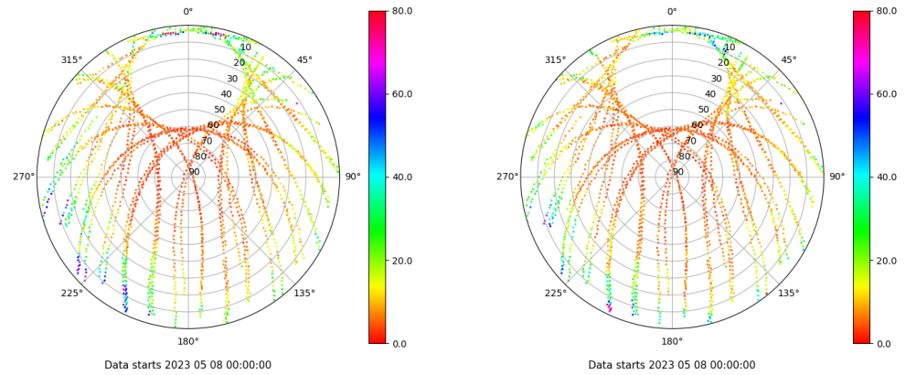
Skyplot for station XIXO. Parameter M1C Data file XIXO00ESP_R_2023128.xtr Skyplot for station XIXO. Parameter M2C Data file XIXO00ESP_R_2023128.xtr
