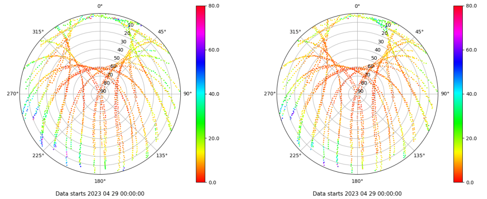
Skyplot for station XIXO. Parameter M1C Data file XIXO00ESP_R_2023119.xtr Skyplot for station XIXO. Parameter M2C Data file XIXO00ESP_R_2023119.xtr
