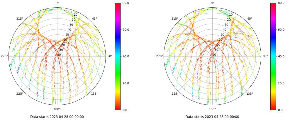
Skyplot for station XIXO. Parameter M1C Data file XIXO00ESP_R_2023118.xtr Skyplot for station XIXO. Parameter M2C Data file XIXO00ESP_R_2023118.xtr
