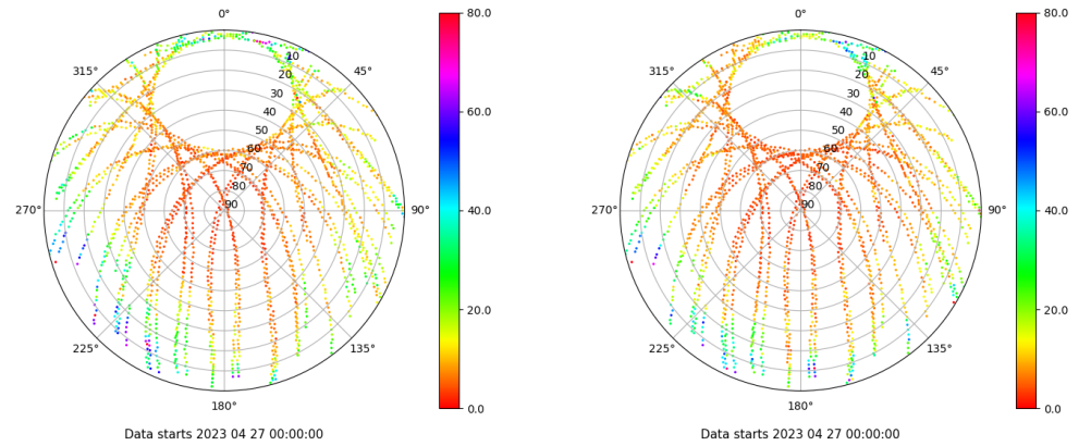
Skyplot for station XIXO. Parameter M1C Data file XIXO00ESP_R_2023117.xtr Skyplot for station XIXO. Parameter M2C Data file XIXO00ESP_R_2023117.xtr
