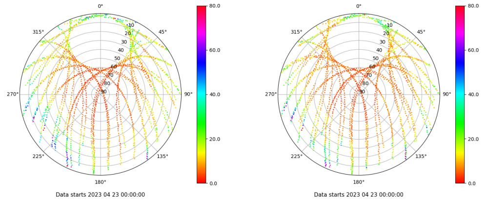
Skyplot for station XIXO. Parameter M1C Data file XIXO00ESP_R_2023113.xtr Skyplot for station XIXO. Parameter M2C Data file XIXO00ESP_R_2023113.xtr
