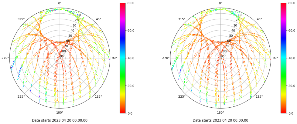
Skyplot for station XIXO. Parameter M1C Data file XIXO00ESP_R_2023110.xtr Skyplot for station XIXO. Parameter M2C Data file XIXO00ESP_R_2023110.xtr
