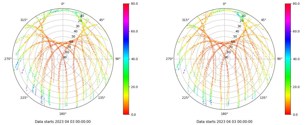
Skyplot for station XIXO. Parameter M1C Data file XIXO00ESP_R_2023093.xtr Skyplot for station XIXO. Parameter M2C Data file XIXO00ESP_R_2023093.xtr
