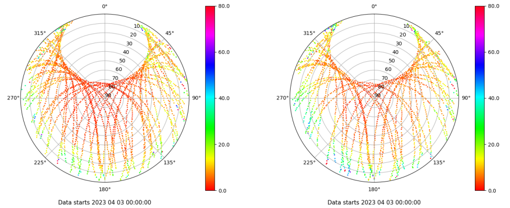
Skyplot for station XIXO. Parameter M1C Data file XIXO00ESP_R_2023093.xtr Skyplot for station XIXO. Parameter M2S Data file XIXO00ESP_R_2023093.xtr
