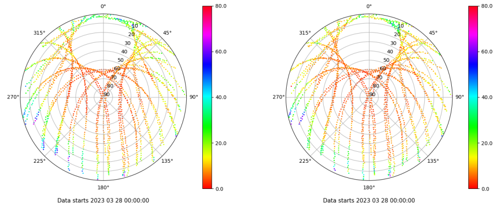
Skyplot for station XIXO. Parameter M1C Data file XIXO00ESP_R_2023087.xtr Skyplot for station XIXO. Parameter M2C Data file XIXO00ESP_R_2023087.xtr
