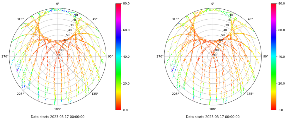
Skyplot for station XIXO. Parameter M1C Data file XIXO00ESP_R_2023076.xtr Skyplot for station XIXO. Parameter M2C Data file XIXO00ESP_R_2023076.xtr
