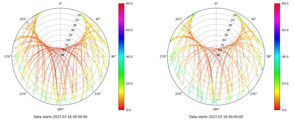
Skyplot for station XIXO. Parameter M1C Data file XIXO00ESP_R_2023075.xtr Skyplot for station XIXO. Parameter M2S Data file XIXO00ESP_R_2023075.xtr
