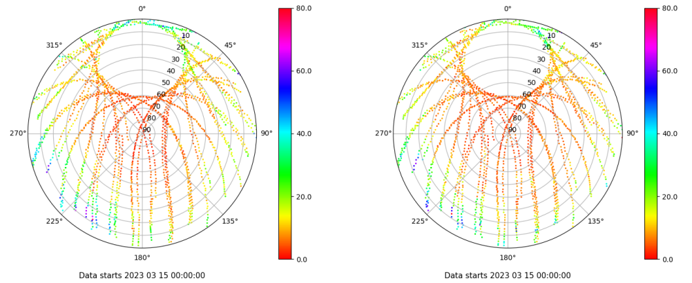
Skyplot for station XIXO. Parameter M1C Data file XIXO00ESP_R_2023074.xtr Skyplot for station XIXO. Parameter M2C Data file XIXO00ESP_R_2023074.xtr
