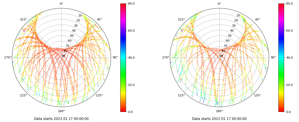
Skyplot for station XIXO. Parameter M1C Data file XIXO00ESP_R_2023017.xtr Skyplot for station XIXO. Parameter M2S Data file XIXO00ESP_R_2023017.xtr
