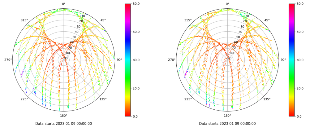
Skyplot for station XIXO. Parameter M1C Data file XIXO00ESP_R_2023009.xtr Skyplot for station XIXO. Parameter M2C Data file XIXO00ESP_R_2023009.xtr
