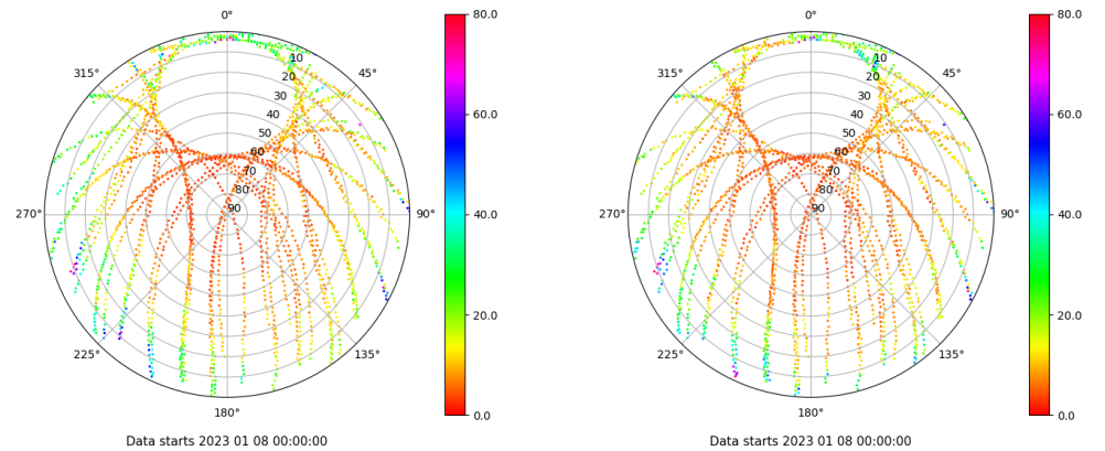
Skyplot for station XIXO. Parameter M1C Data file XIXO00ESP_R_2023008.xtr Skyplot for station XIXO. Parameter M2C Data file XIXO00ESP_R_2023008.xtr
