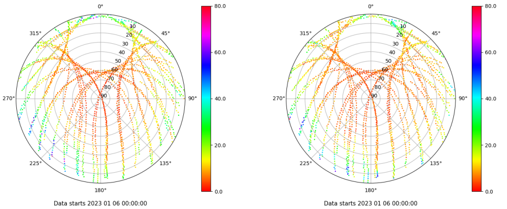
Skyplot for station XIXO. Parameter M1C Data file XIXO00ESP_R_2023006.xtr Skyplot for station XIXO. Parameter M2C Data file XIXO00ESP_R_2023006.xtr
