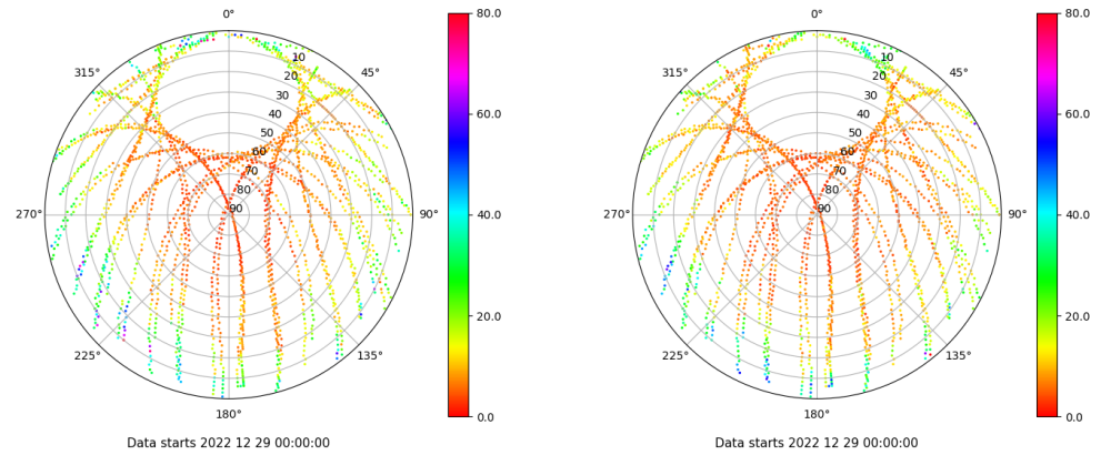
Skyplot for station XIXO. Parameter M1C Data file XIXO00ESP_R_2022363.xtr Skyplot for station XIXO. Parameter M2C Data file XIXO00ESP_R_2022363.xtr
