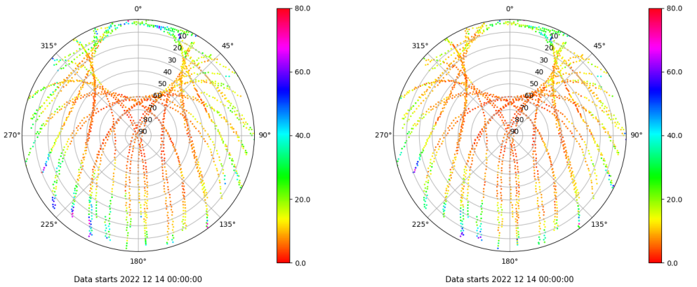
Skyplot for station XIXO. Parameter M1C Data file XIXO00ESP_R_2022348.xtr Skyplot for station XIXO. Parameter M2C Data file XIXO00ESP_R_2022348.xtr
