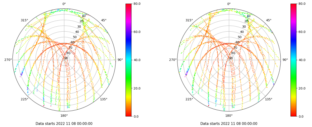
Skyplot for station XIXO. Parameter M1C Data file XIXO00ESP_R_2022312.xtr Skyplot for station XIXO. Parameter M2C Data file XIXO00ESP_R_2022312.xtr
