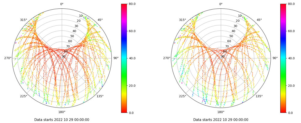
Skyplot for station XIXO. Parameter M1C Data file XIXO00ESP_R_2022302.xtr Skyplot for station XIXO. Parameter M2S Data file XIXO00ESP_R_2022302.xtr
