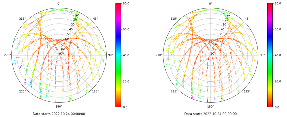
Skyplot for station XIXO. Parameter M1C Data file XIXO00ESP_R_2022297.xtr Skyplot for station XIXO. Parameter M2C Data file XIXO00ESP_R_2022297.xtr
