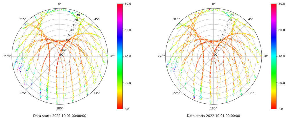
Skyplot for station XIXO. Parameter M1C Data file XIXO00ESP_R_2022274.xtr Skyplot for station XIXO. Parameter M2C Data file XIXO00ESP_R_2022274.xtr
