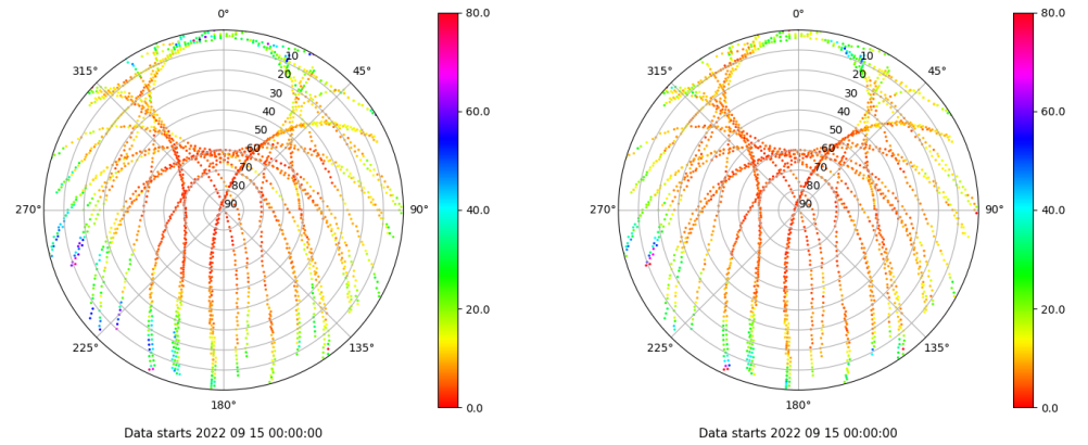
Skyplot for station XIXO. Parameter M1C Data file XIXO00ESP_R_2022258.xtr Skyplot for station XIXO. Parameter M2C Data file XIXO00ESP_R_2022258.xtr
