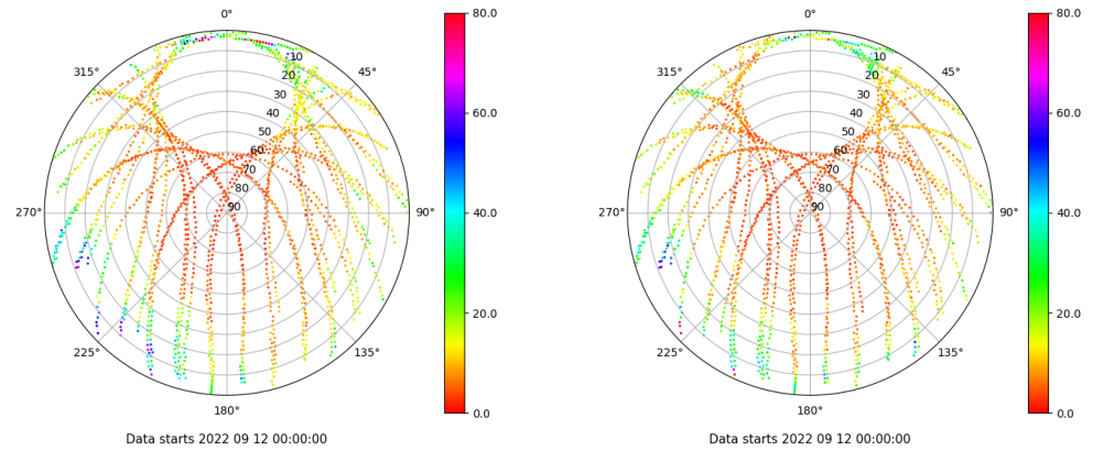
Skyplot for station XIXO. Parameter M1C Data file XIXO00ESP_R_2022255.xtr Skyplot for station XIXO. Parameter M2C Data file XIXO00ESP_R_2022255.xtr
