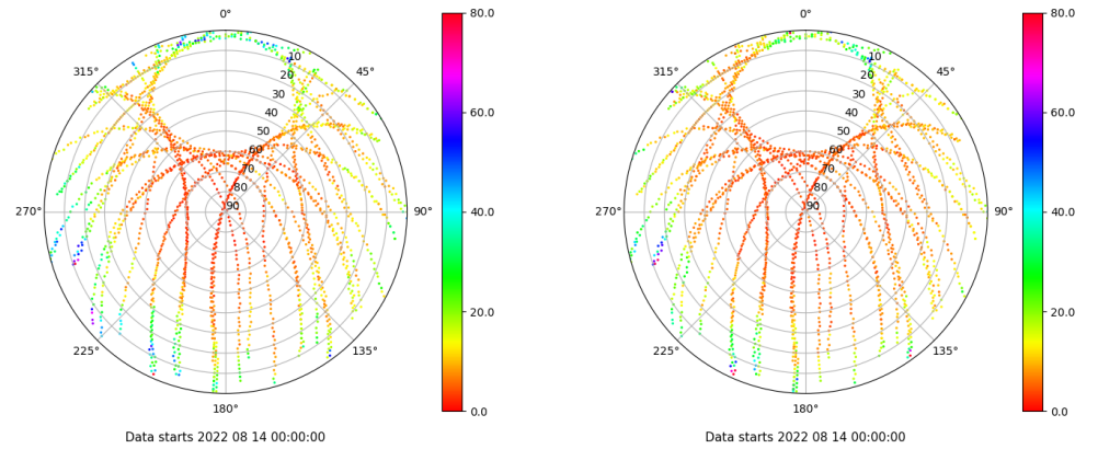
Skyplot for station XIXO. Parameter M1C Data file XIXO00ESP_R_2022226.xtr Skyplot for station XIXO. Parameter M2C Data file XIXO00ESP_R_2022226.xtr
