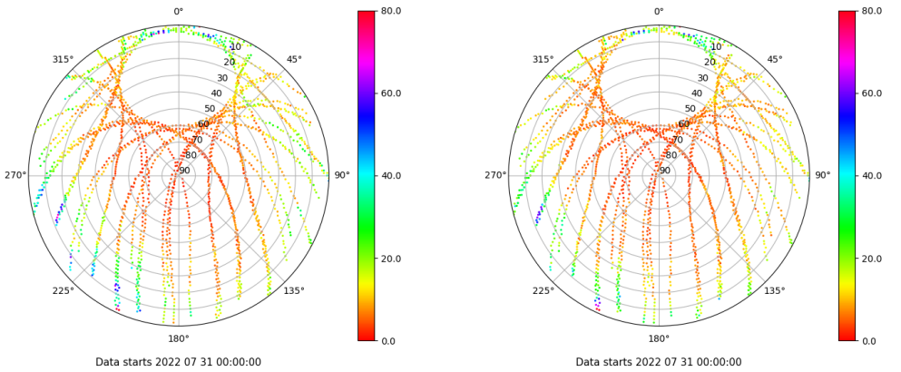
Skyplot for station XIXO. Parameter M1C Data file XIXO00ESP_R_2022212.xtr Skyplot for station XIXO. Parameter M2C Data file XIXO00ESP_R_2022212.xtr
