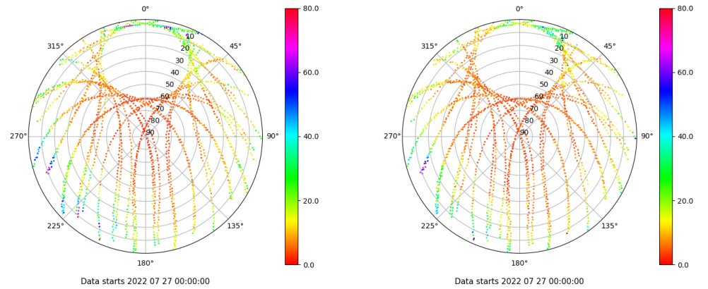
Skyplot for station XIXO. Parameter M1C Data file XIXO00ESP_R_2022208.xtr Skyplot for station XIXO. Parameter M2C Data file XIXO00ESP_R_2022208.xtr
