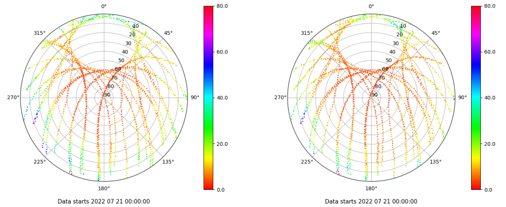
Skyplot for station XIXO. Parameter M1C Data file XIXO00ESP_R_2022202.xtr Skyplot for station XIXO. Parameter M2C Data file XIXO00ESP_R_2022202.xtr
