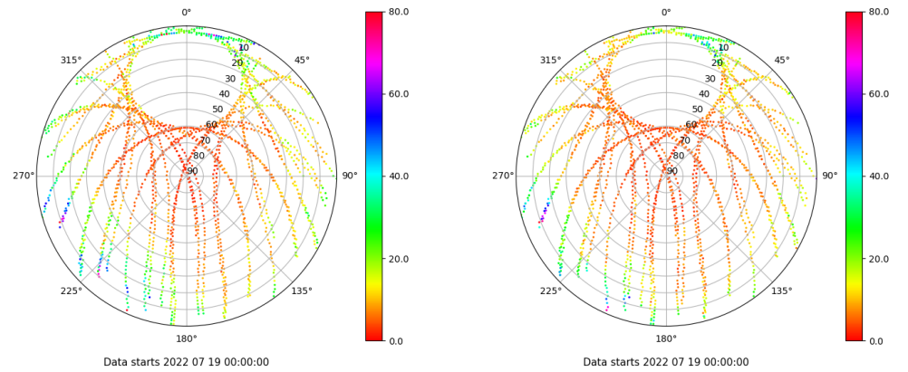
Skyplot for station XIXO. Parameter M1C Data file XIXO00ESP_R_2022200.xtr Skyplot for station XIXO. Parameter M2C Data file XIXO00ESP_R_2022200.xtr
