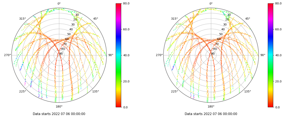
Skyplot for station XIXO. Parameter M1C Data file XIXO00ESP_R_2022187.xtr Skyplot for station XIXO. Parameter M2C Data file XIXO00ESP_R_2022187.xtr
